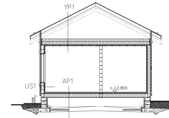
leikkaus A-A
