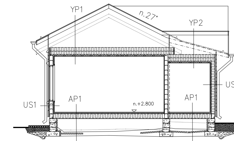
leikkaus B-B
