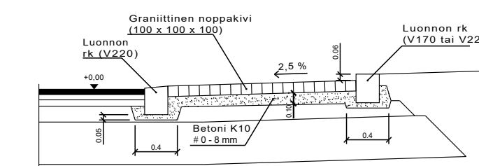
KIERTOTILAN KAVENNUKSEN LEIKKAUS, A - A, (1:50)
